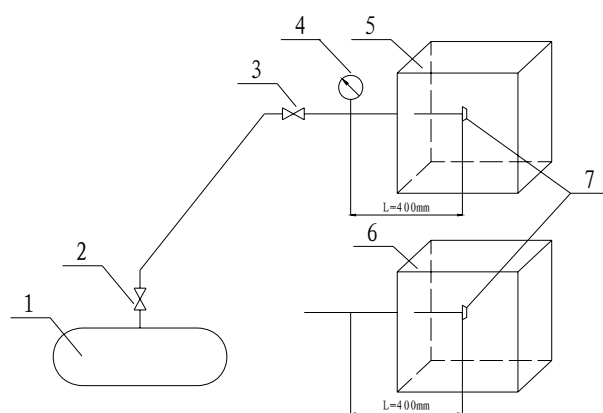
图4 喷嘴耐热和耐压试验装置
