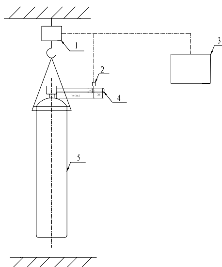
图 3a) 喷嘴流量特性试验装置原理示意图 (重量平衡方式)
