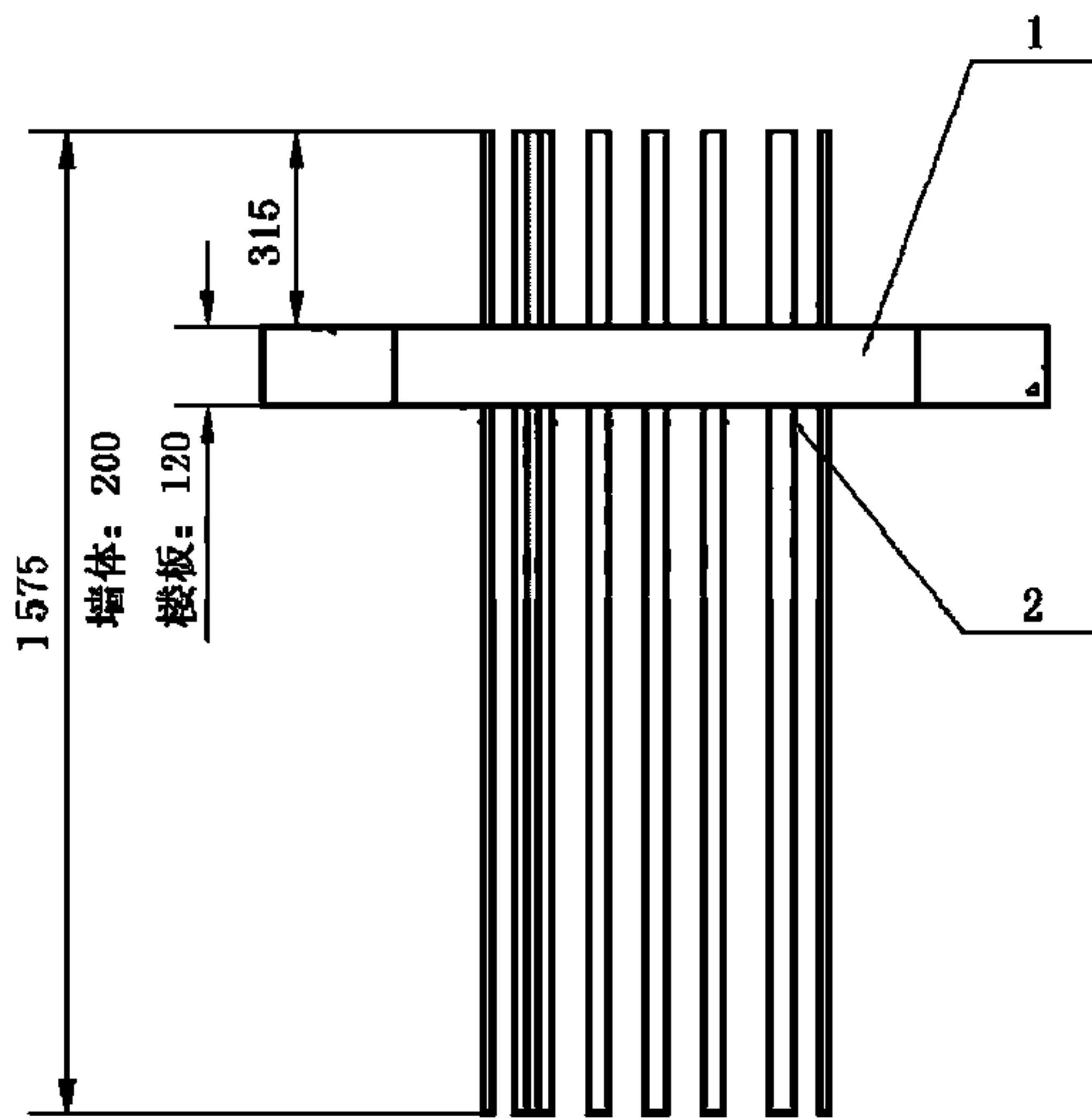
俯视图
