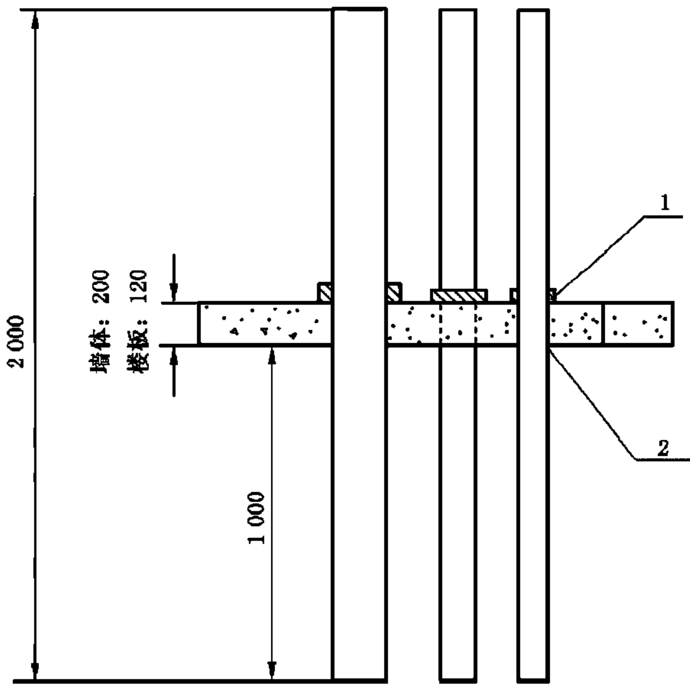
A—A 剖面图
