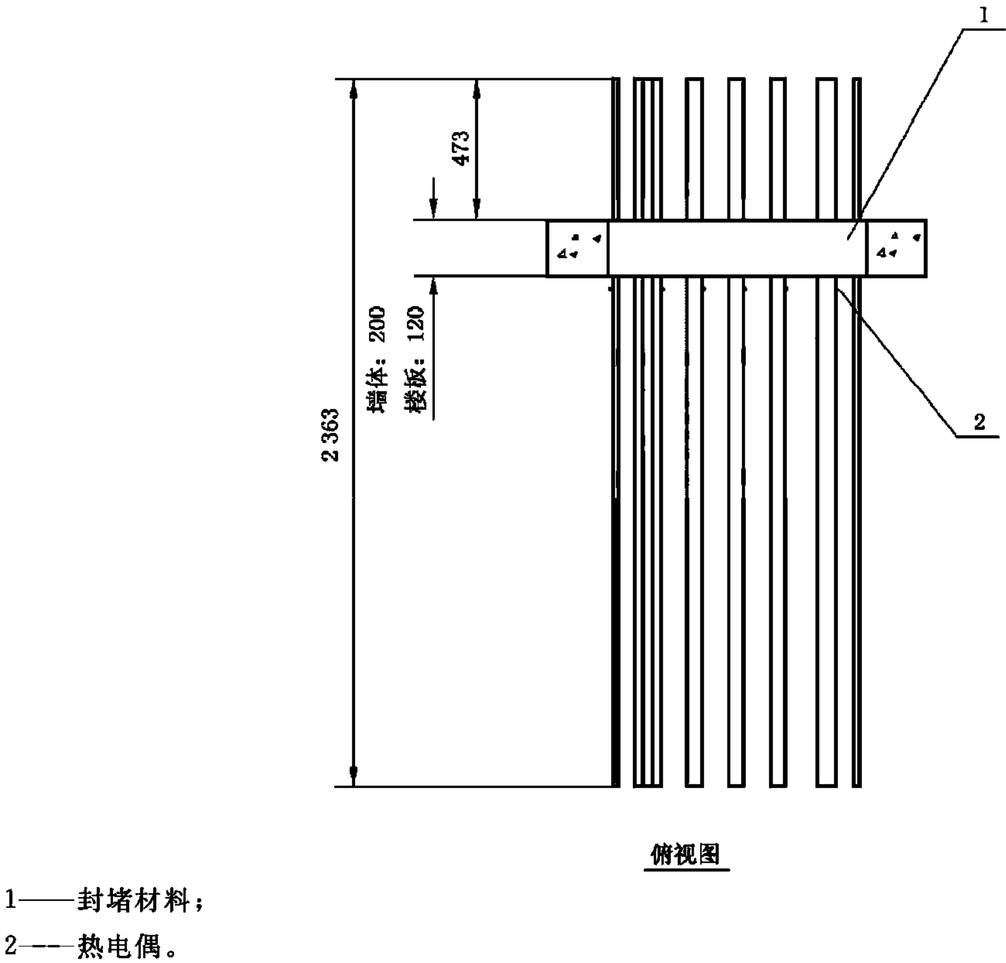
图 A.2 柔性有机堵料、泡沫封堵材料电缆贯穿标准试件的安装方式
