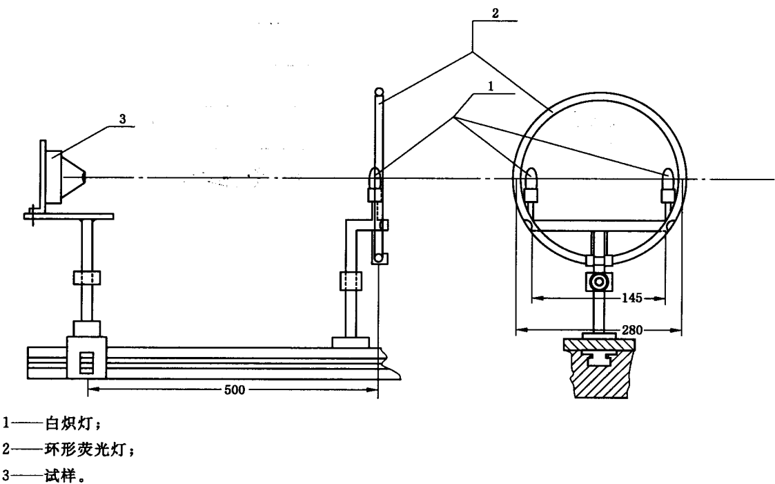
图 5 环境光干扰试验装置结构图
