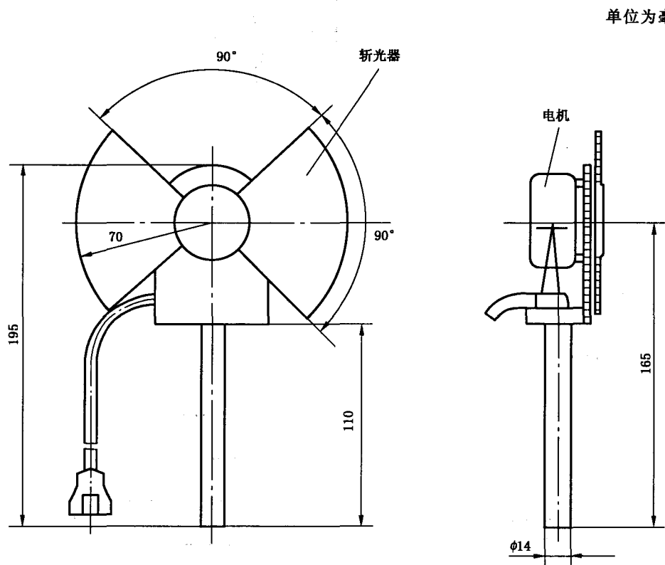
图 2 调制器结构图
