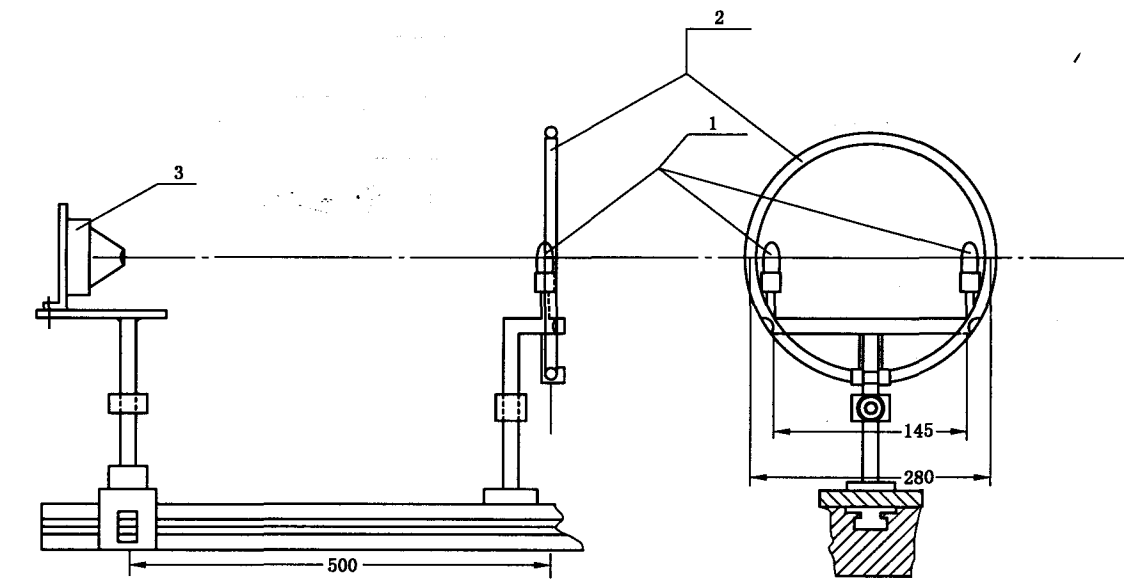
1——白炽灯； 2——环形荧光灯； 3——试样。
